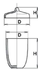
Kelímek pro stanovení prchavé kapaliny s víčkem Crucible for determination of volatile liquid with lid Tiegel für Festsetzung vergängliche Flüssigkeit mit Deckel Crisol con tapa para prefinción de fluido disipable Тигель для определения летучей жидкости с крышкой
